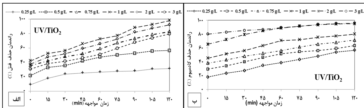
شکل شماره ۲. تاثیر مقدار نانوذرات بر کارایی حذف فنل (الف) ( pH=7, Cd=5mg/L, Phenol=15mg/L ) و زمان 120min (ب) و کادمیوم ( Phenol=5mg/L, Cd=15mg/L ) توسط فرآیند UV/TiO_2 در مدت زمان واکنش مشخص
