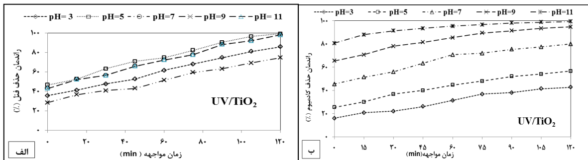
شکل شماره ۳. تاثیر pH بر کارایی حذف فنل (الف) ( Phenol=15 \text{ mg/L} , Cd=5 \text{ mg/L} , دوز TiO_2=1 \text{ g/L} و 120 \text{ min} زمان مواجهه) و کادمیوم (ب) ( Phenol=5 \text{ mg/L} , Cd=15 \text{ mg/L} ) توسط فرآیند UV/TiO_2 در مدت زمان واکنش مشخص
