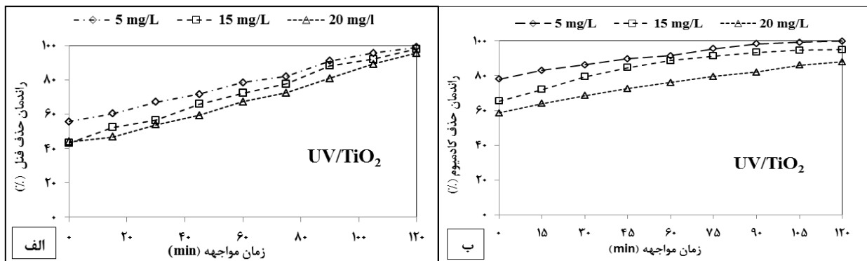
شکل شماره ۴. تاثیر غلظت اولیه بر کارایی حذف فنل (الف) ( pH=7 , Cd=5 \text{ mg/L} , دوز TiO_2=1 \text{ g/L} و 120 \text{ min} زمان مواجهه) و کادمیوم (ب) ( pH=7 , phenol=5 \text{ mg/L} , دوز TiO_2=2 \text{ g/L} ) بر کارایی حذف فنل توسط فرآیند UV/TiO_2 در مدت زمان واکنش مشخص
