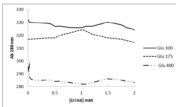
شکل شماره ۲. جذب طول موج ۲۸۰ نانومتر آلبومین سرم انسانی در حضور غلظت های مختلف گلوکز در دمای ۴۲ درجه سانتی گراد به عنوان تابعی از غلظت DTAB در بافر فسفات نیم میلی مولار و pH=7
