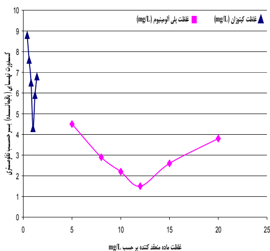
شکل شماره ۴. کارایی حذف کدورت در انواع و غلظت های مختلف منعقد کننده در کدورت اولیه ۵۰۰ واحد نفلومتری
