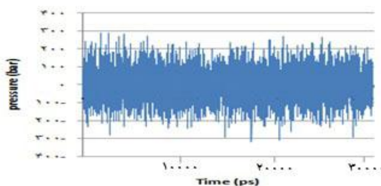
نمودار شماره ۲. نمودار تغییرات فشار آنزیم سیکلو اکسیژناز ۲
