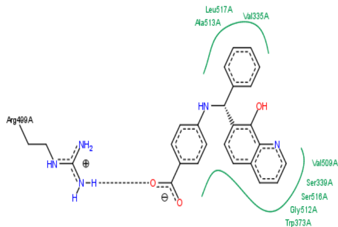
شکل شماره ۱. نمایی از برهمکنش آنزیم سیکلواکسیژناز ۲ با مهارکننده شماره ۶۴۳۷۳۵ (بهترین لیگاند) در جایگاه فعال آنزیم
