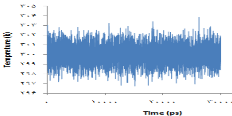
نمودار شماره ۱. نمودار تغییرات دمایی آنزیم سیکلو اکسیژناز ۲
