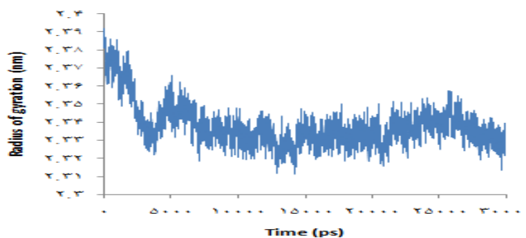
نمودار شماره ۳. نمودار شعاع ژیراسیون آنزیم سیکلو اکسیژناز ۲
