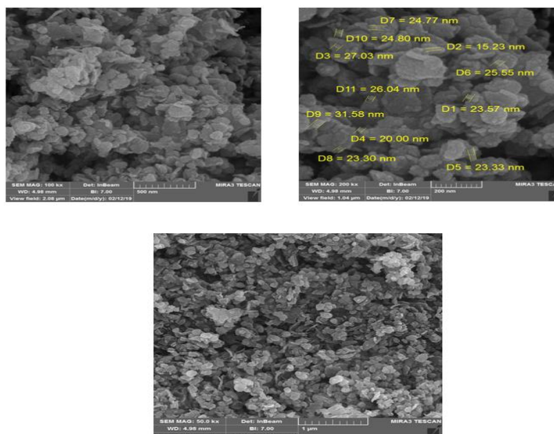
شکل شماره ۱. تصاویر میکروسکوپی (FESEM) نانوذرات اکسیدروی سنتز شده توسط مواد درون سلولی مخمر
