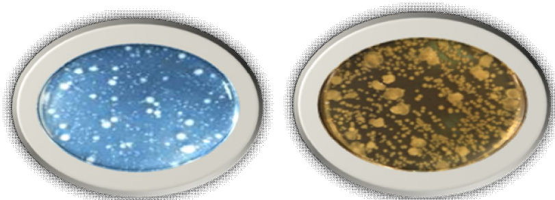
شکل شماره ۳. کلنی باکتریها و قارچ های رشد کرده بر روی سطح پلیت در حالت بیشترین PM_{10} (سمت چپ) و کمترین PM_{10} (سمت راست) بر حسب میکروگرم در مترمکعب
