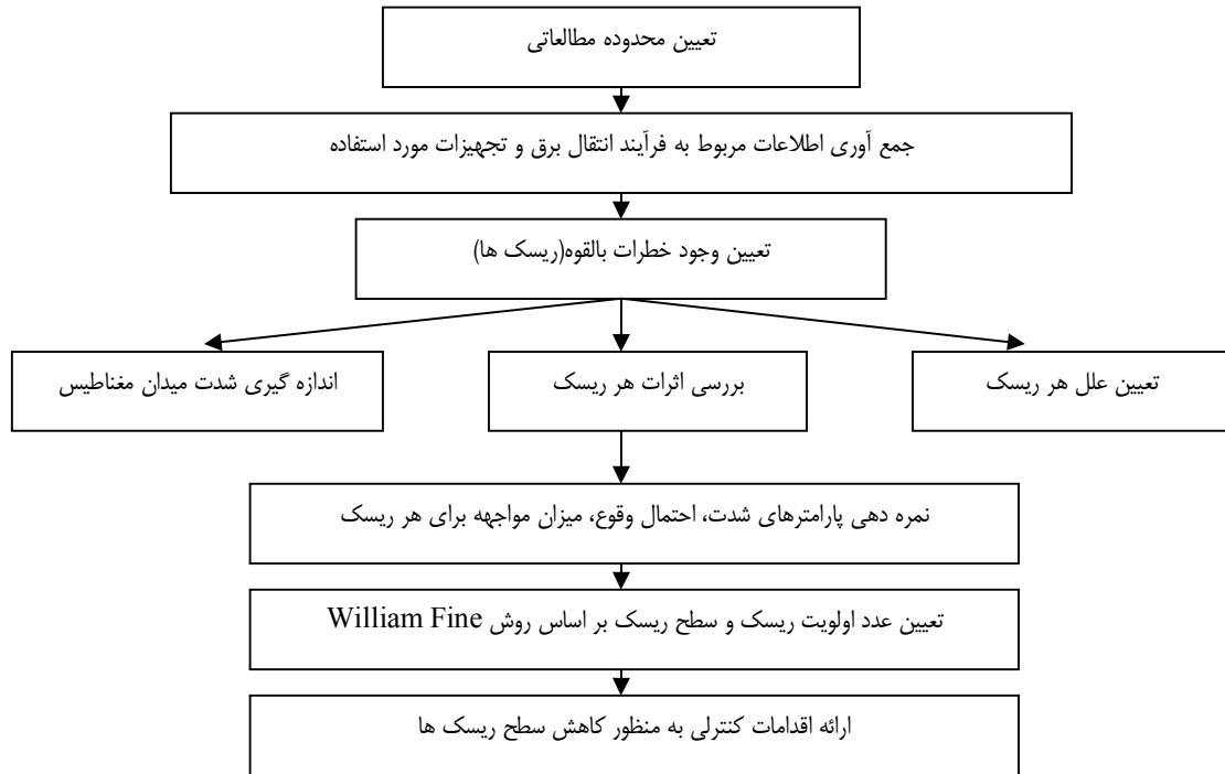
نمودار شماره ۱. مراحل انجام ارزیابی ریسک خطوط انتقال برق منطقه حصارآباد اهواز
