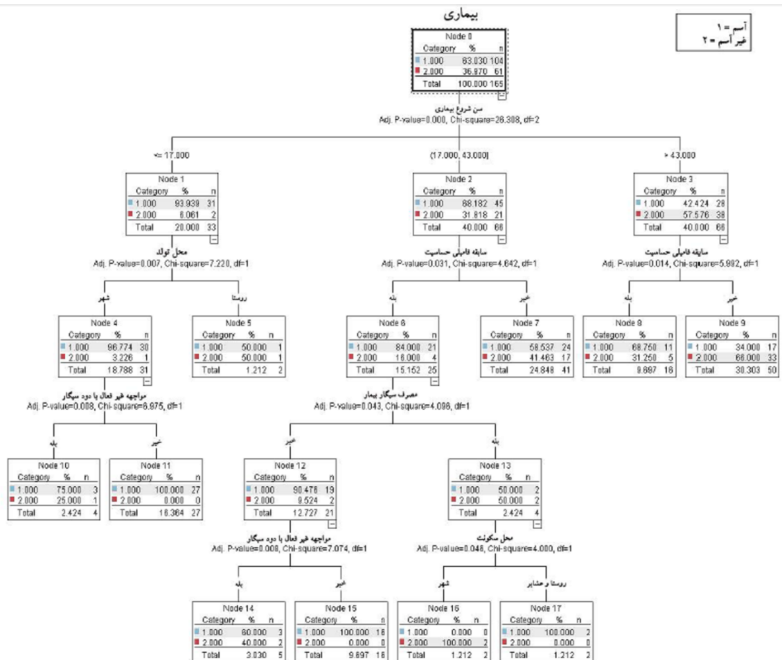
شکل شماره ۱. مدل ایجاد شده توسط الگوریتم CHAID
