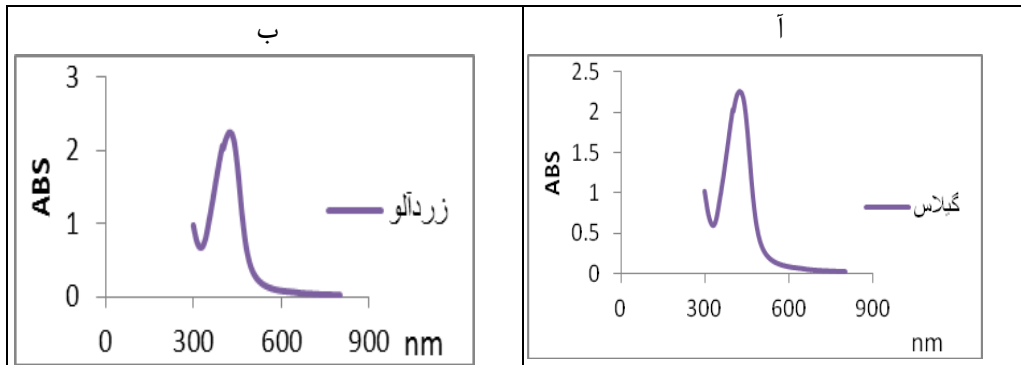
شکل شماره ۲. میزان جذب نانوذرات نقره. نانوذرات نقره سنتز شده از صمغ درخت گیلاس (آ) و زردآلو (ب) با استفاده از دستگاه اسپکتروفوتومتر UV-Vis از طول موج ۳۰۰ تا ۸۰۰ نانومتر.
