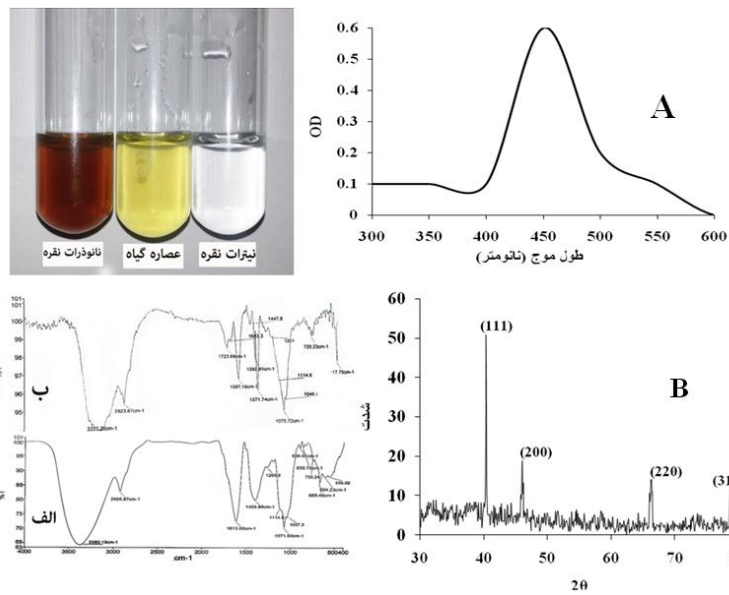
شکل شماره ۱- A: طیف UV/Visible مخلوط واکنش (نیترات نقره ۱ میلی مولار و عصاره در غلظت ۱ میلی گرم بر میلی لیتر) از زرد به قهوه ای در دمای ۲۰ درجه سانتی گراد. B: تصویر پراش X-ray مربوط به نانوذرات نقره سنتز شده توسط عصاره بذر و طیف مادون قرمز (FTIR) عصاره الف: قبل از واکنش، ب: پس از واکنش
