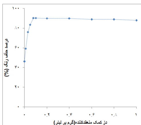
شکل شماره 2. تاثیر دز کمک منعقد کننده بر کارایی حذف رنگ دیسپرس رد 60
